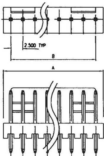
Lötanschluss direkt
