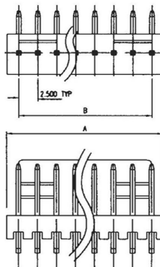
Lötanschluss 90°
