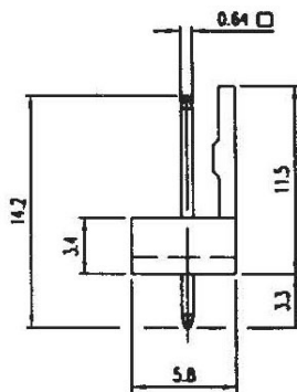
Lötanschluss direkt
